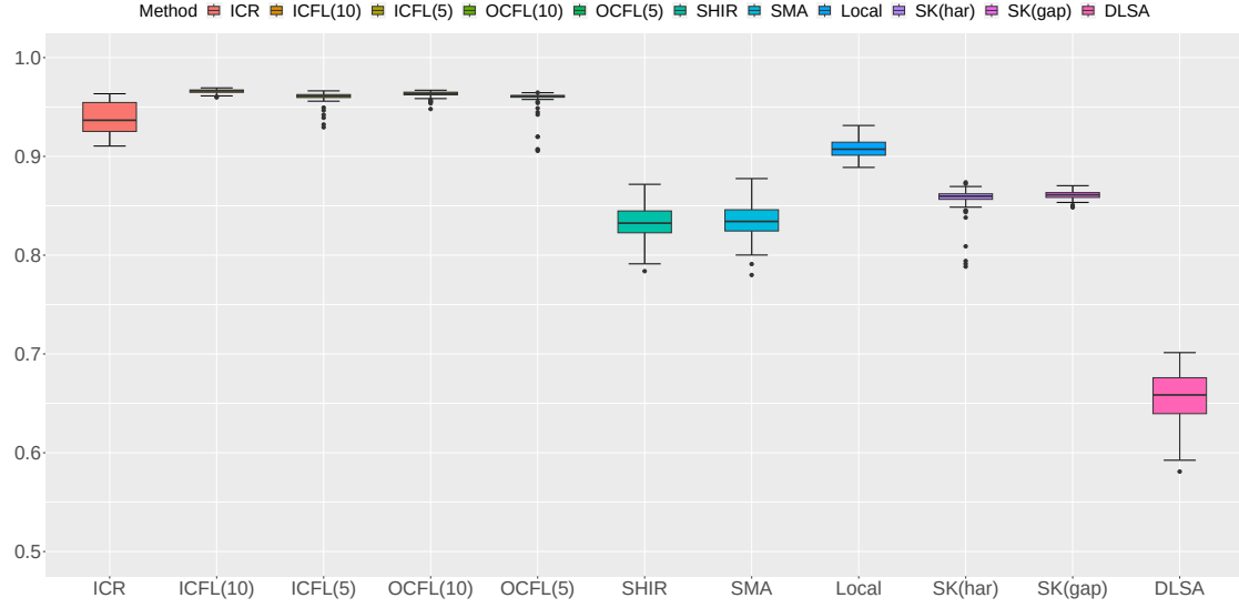
(a) AUC
